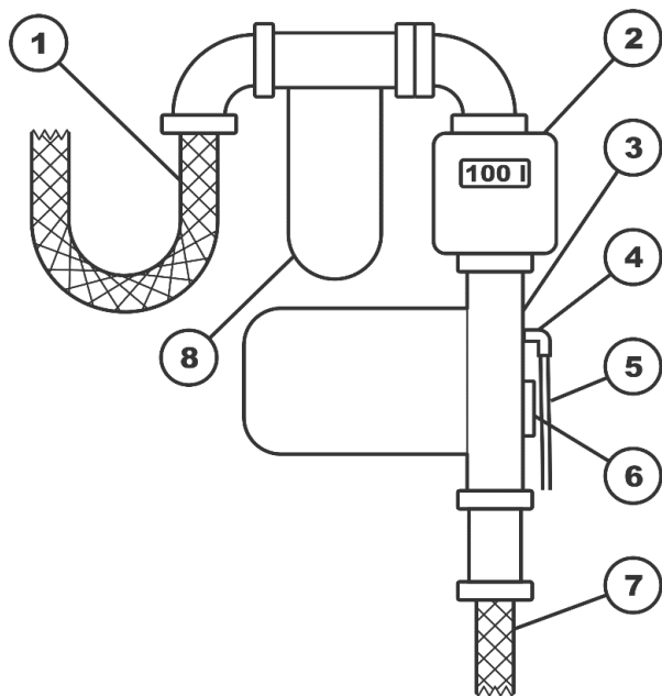
Schemat układu dystrybucyjnego
