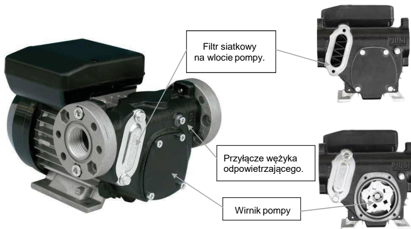
Pompa Panther firmy PIUSI
